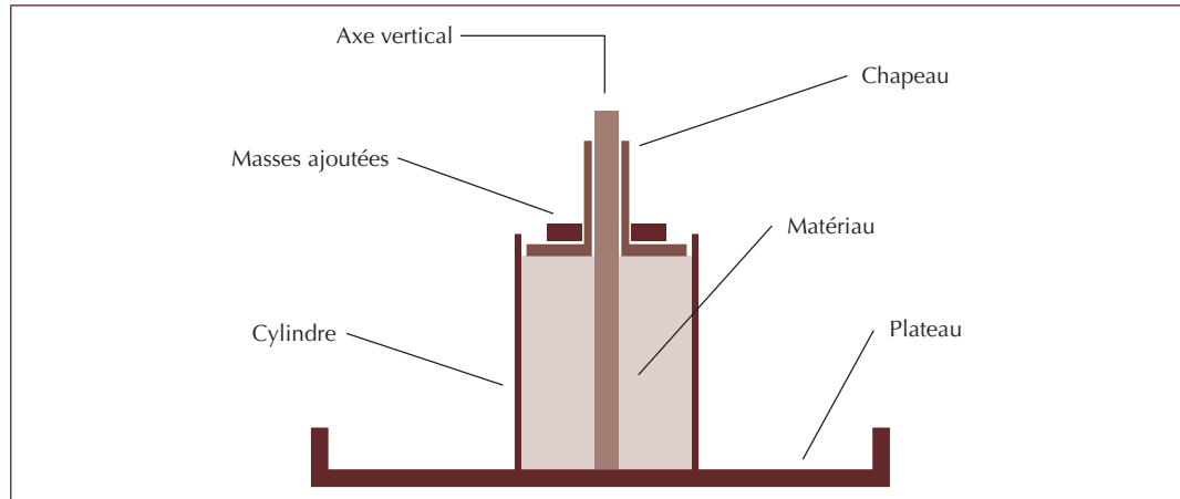
► Figure 1-a – Schéma du slump-test .
