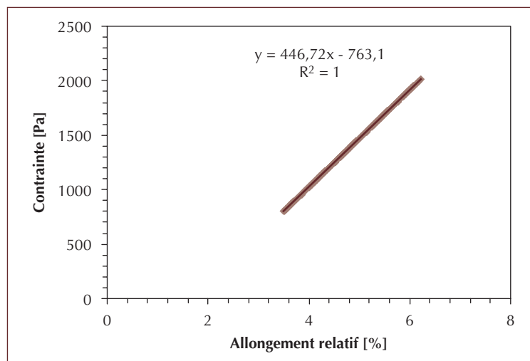
▲ Figure 1-c – Détermination du module élastique, pour la boue issue du lit F.
